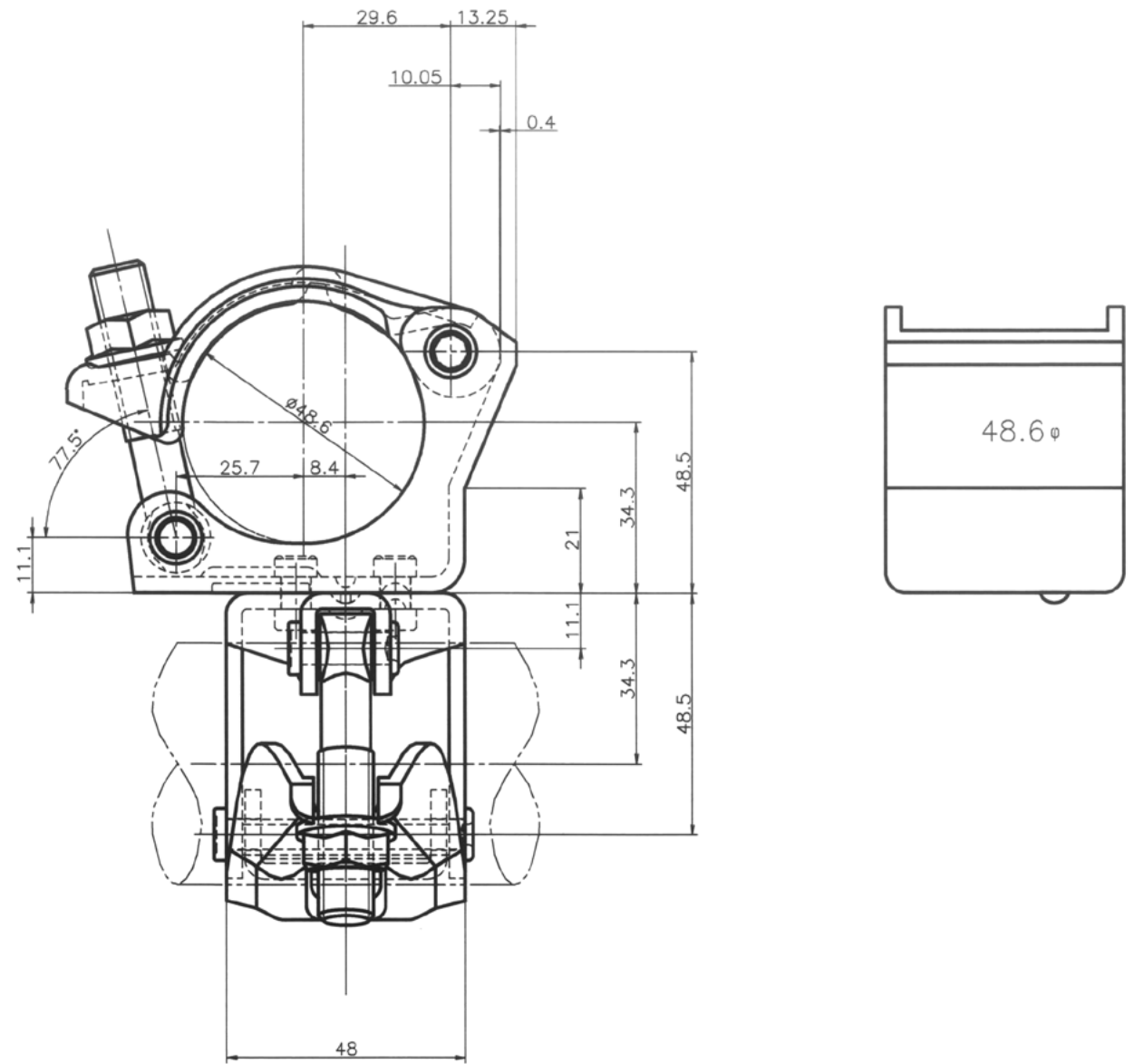
Ø48.6同径ALLドブメッキランプ (直交型)
