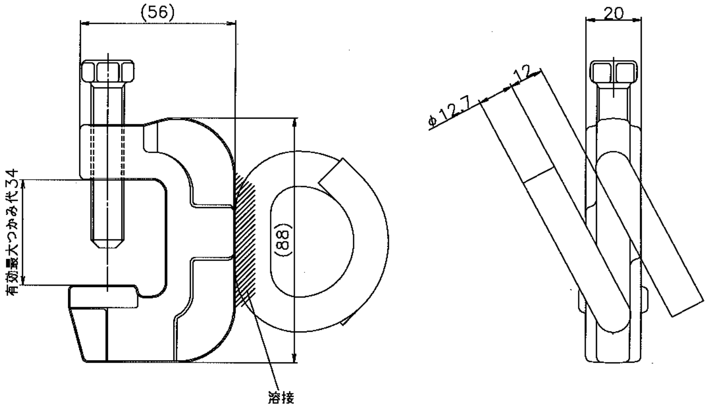
ネット用クランプ
