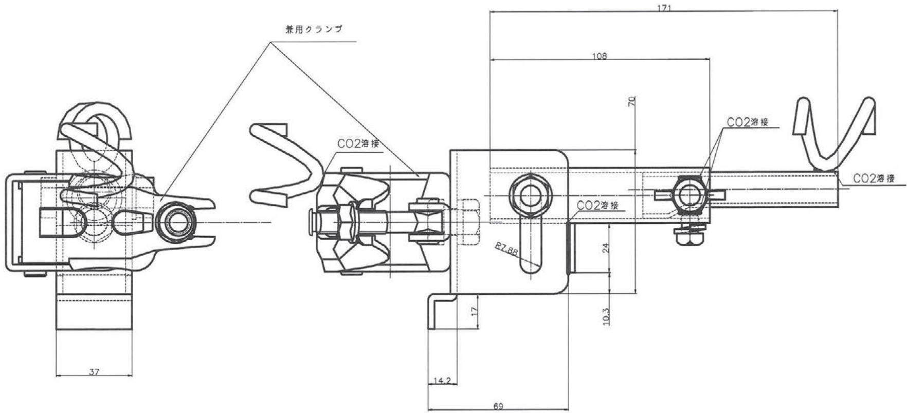
ASB-3T スマートブラケット
